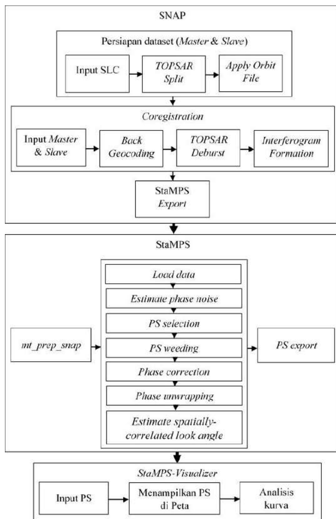
Gambar 2.3 Tahapan pengolahan data PSInSAR di lapangan panas bumi Ulubelu
