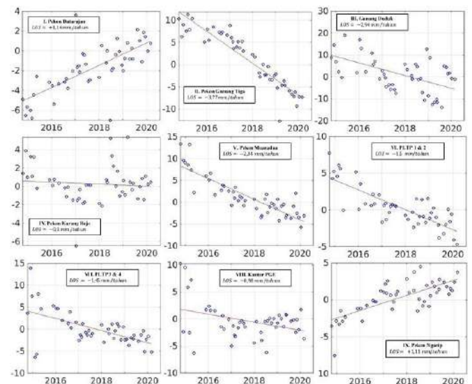
Gambar 3.6 Kurva laju deformasi LOS tiap area vital di wilayah panas bumi Ulubelu
