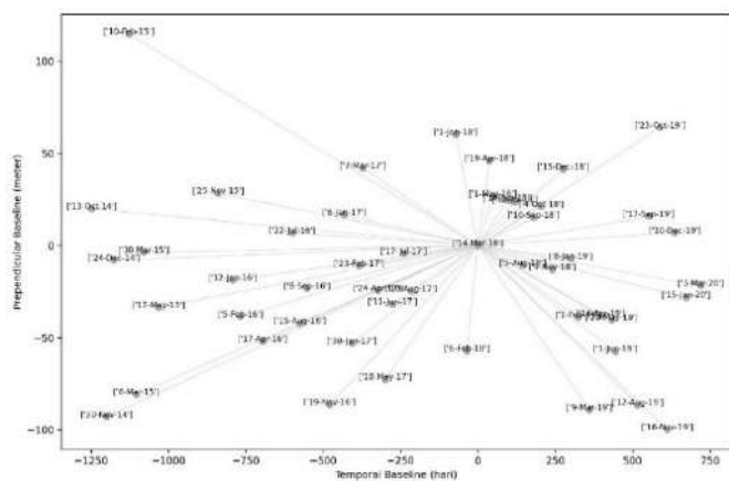
Gambar 2.2 Grafik hubungan perpendicular baseline dan temporal baseline data InSAR
