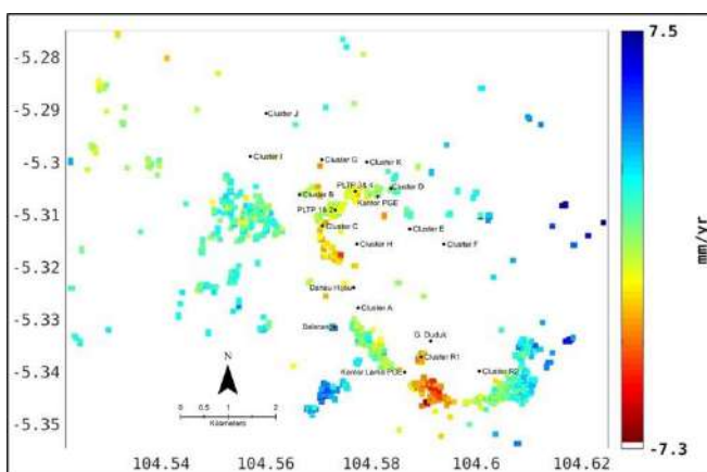
Gambar 3.2 Peta laju deformasi rata-rata (mm/tahun) di area panas bumi Ulubelu
