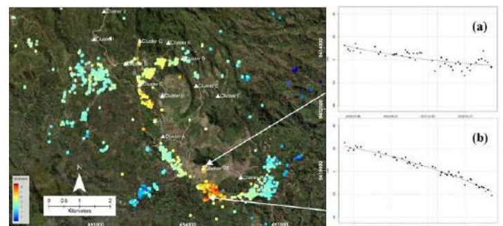
Gambar 3.3 Peta dan kurva laju deformasi di area Gunung Duduk (a) dan Pekon Gunung Tiga (b) lapangan panas bumi Ulubelu. Lokasi titik PS ditunjukkan oleh panah berwarna putih pada gambar.
