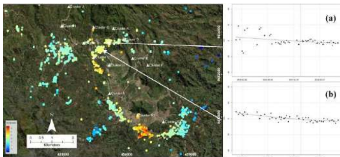
Gambar 3.4 Peta dan kurva laju deformasi di area PLTP unit 3 & 4 (a) dan PLTP unit 1 & 2 (b) lapangan panas bumi Ulubelu. Lokasi titik PS ditunjukkan oleh panah berwarna putih pada gambar.
