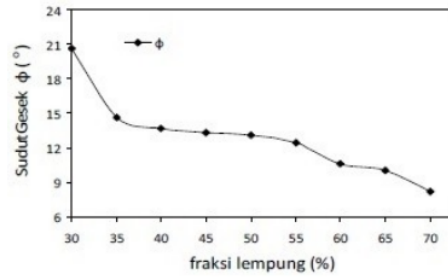
Gambar 1. Hasil uji Direct Shear untuk sudut gesek
