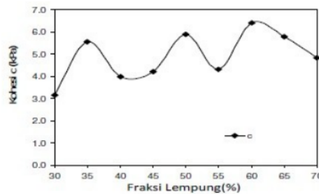
Gambar 3. Hasil uji Direct Shear untuk nilai kohesi
