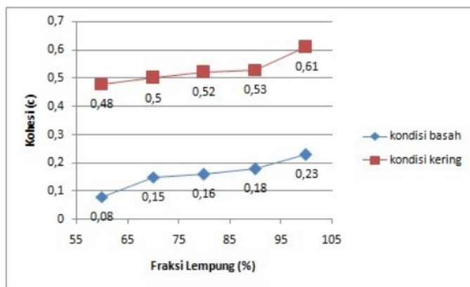
17 Gambar 7. Hubungan fraksi lempung dengan nilai kohesi hasil pengujian geser langsung ( Direct Shear Test ) pada Kondisi Basah dan Kondisi Kering
