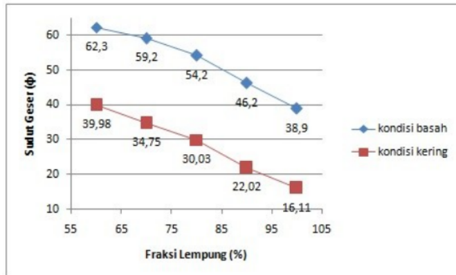
Gambar 8. Hubungan fraksi lempung dengan nilai sudut geser hasil pengujian langsung ( Direct Shear Test ) pada Kondisi Basah dan Kondisi Kering
