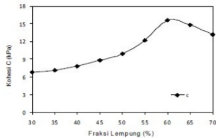
Gambar 4. Hasil uji Triaksial untuk nilai kohesi
