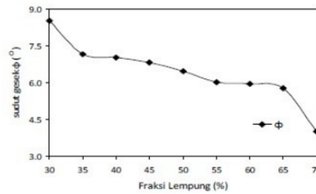
Gambar 2. Hasil uji Triaksial untuk sudut gesek
