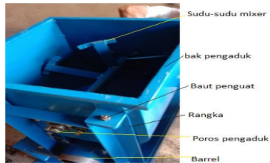
Gambar 2. Bak pengaduk dan pencampur adonan pakan ternak yang akan dicetak pelet
