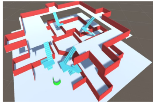
Gambar 10. Visualisasi 3D
