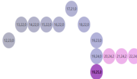
Gambar 9. Visualisasi Pathfinding
