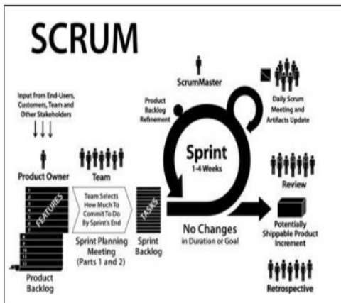
Gambar 2. Artefak pada metode scrum The Scrum Papers (2011).
