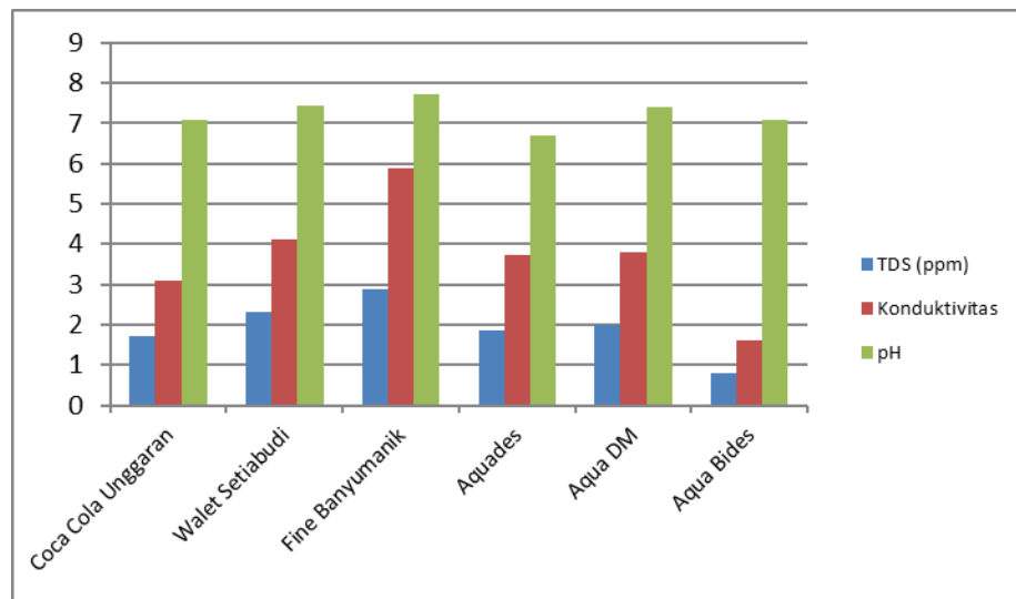
Gambar 1. Diagram perbandingan sampel air AC, Aquades, Aqua DM, dan Aquabides setelah melewati Resin Kation dan Anion .
