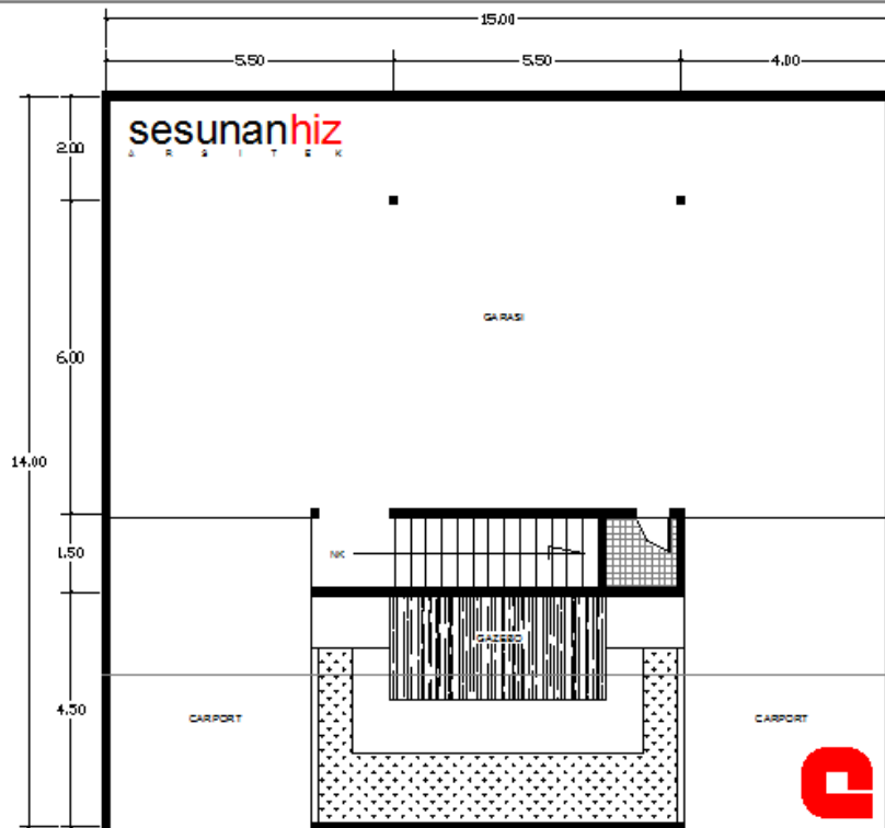
DENAH LT. 1 TANPA SKALA
