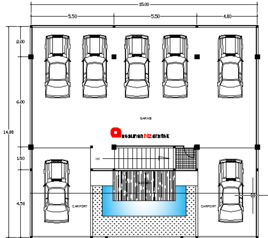
DENAH LT. 1 TANPA SKALA
