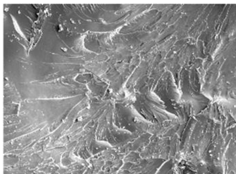
Gambar 4. Permukaan patahan komposit poliester murni
