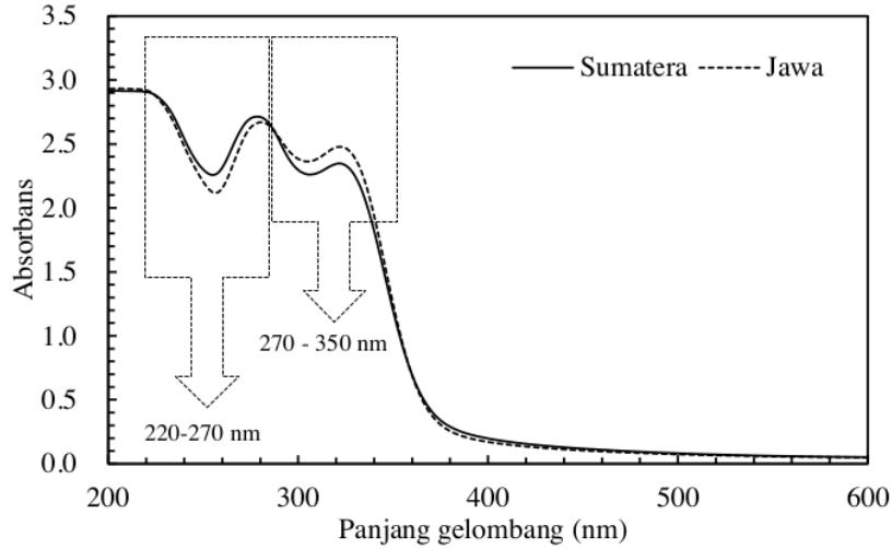
1 Gambar 1. Spektra asli sampel kopi robusta Sumatera dan Jawa pada panjang gelombang 200–600 nm.
