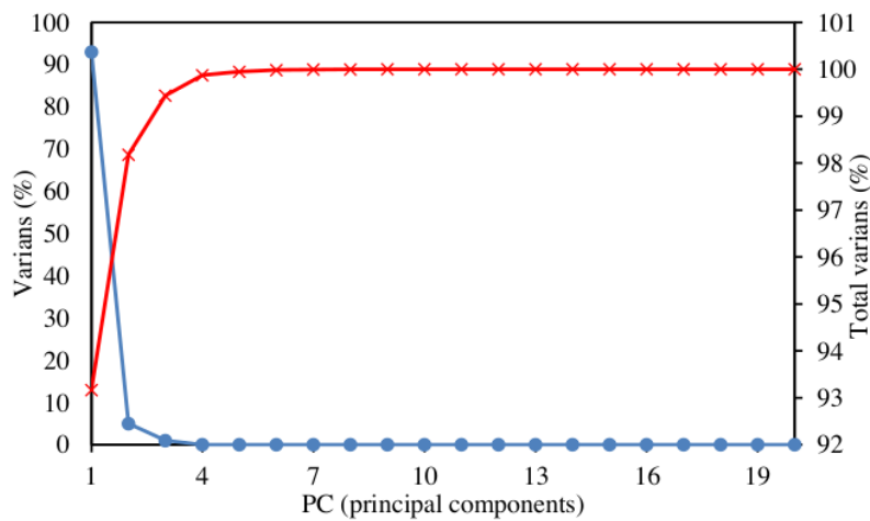
Gambar 2. Hasil plot PCA lengkap dengan nilai variansi dan akumulasinya.
