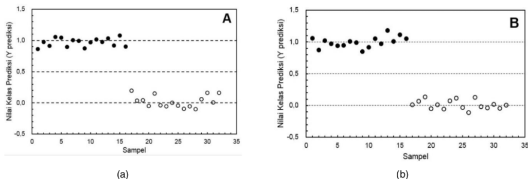
Gambar 6 Hasil prediksi untuk klasifikasi kopi Kalosi (●) dan kopi Toraja (○) menggunakan model PLS-DA spektra hasil transformasi (a) panjang gelombang terpilih 190–1100 nm dan (b) panjang gelombang terpilih 250–450 nm.
