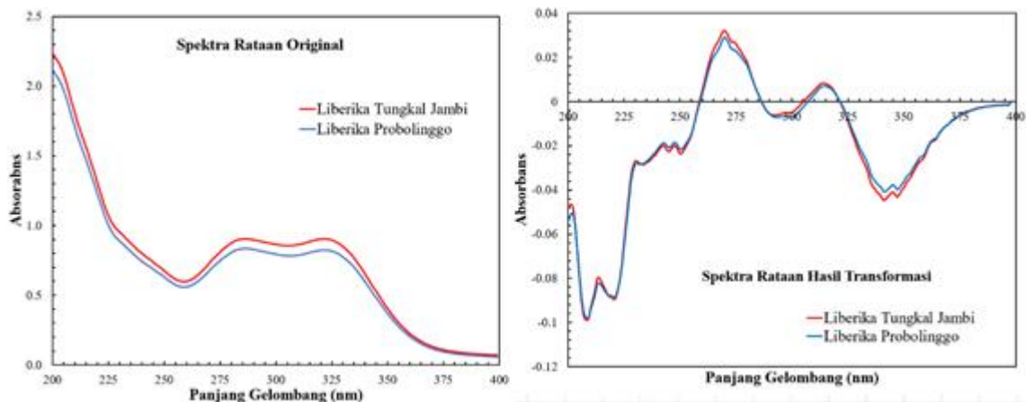
Gambar 2. Spektra Rataan Original dan Hasil Transformasi Sampel Kopi Liberika Tungal Jambi dan Probolinggo di Interval 200-400 nm
