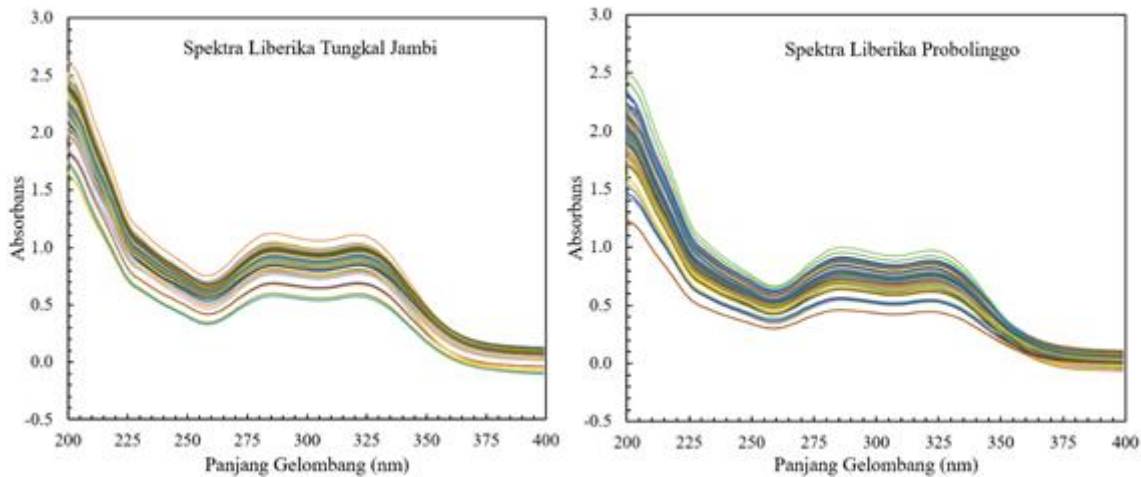
Gambar 1. Spektra Original Sampel Kopi Liberika Tungal Jambi dan Probolinggo di Interval 200-400 nm
