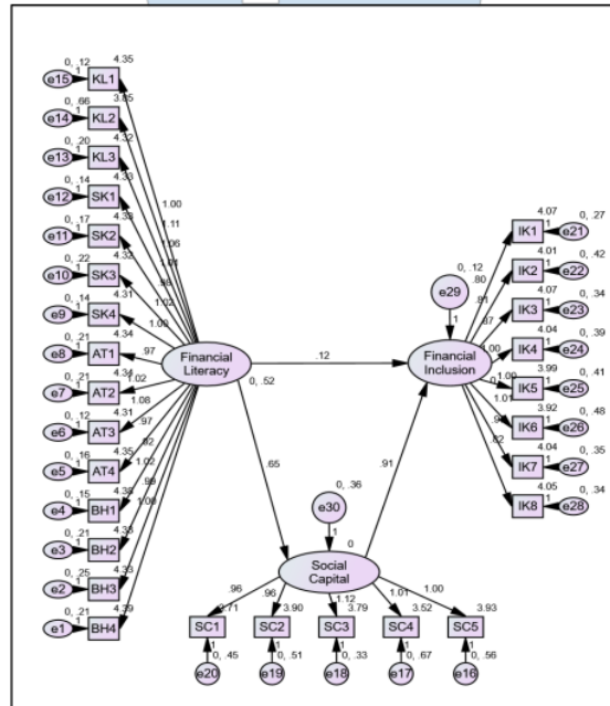
Sumber : Hasil Pengolahan Data Primer (2019) Gambar 2. Model Struktural
