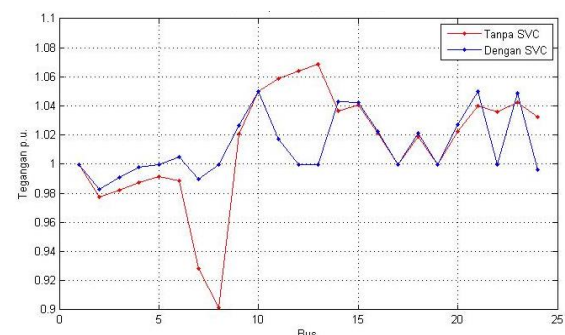
Gambar 7. Grafik Profil Tegangan Sesudah dan Sebelum penempatan SVC pada Bus 8 (Gumawang)
