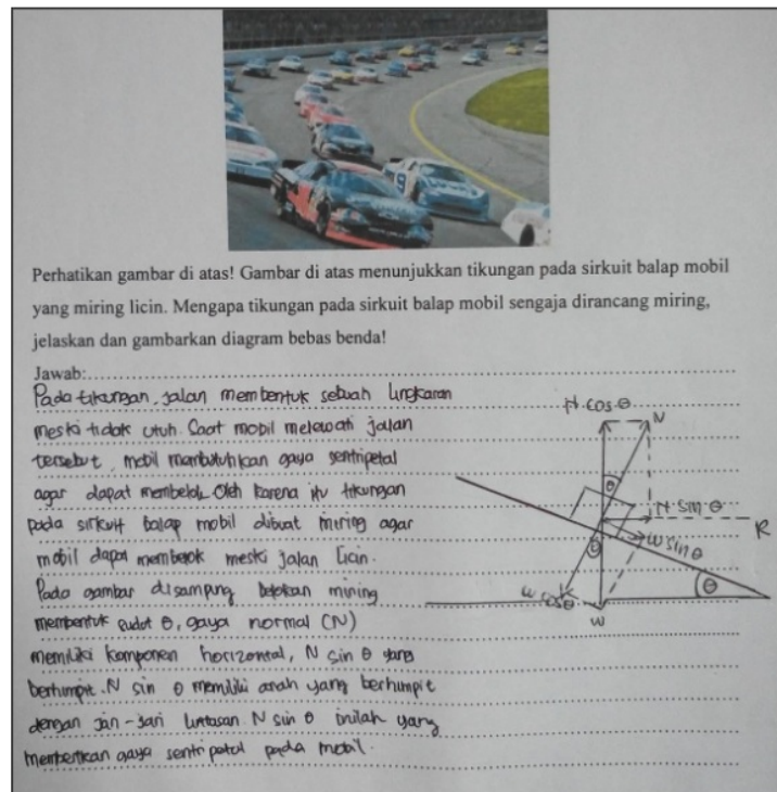
Gambar 5. Analisis Engineering dari Tikungan Miring pada Sirkuit Balap Mobil menggunakan Representasi Verbal, Gambar, dan Matematika
