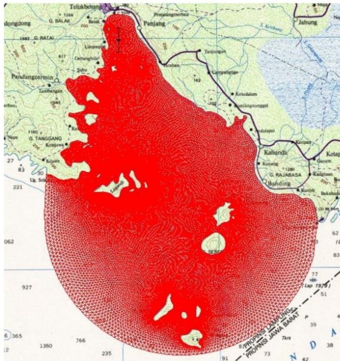
Gambar 7. Mesh modul
