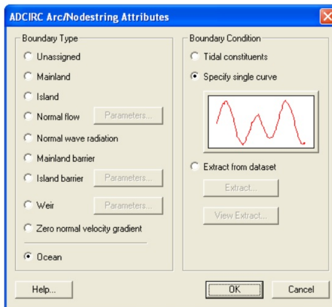
Gambar 8. Pasang surut sebagai kondisi batas
