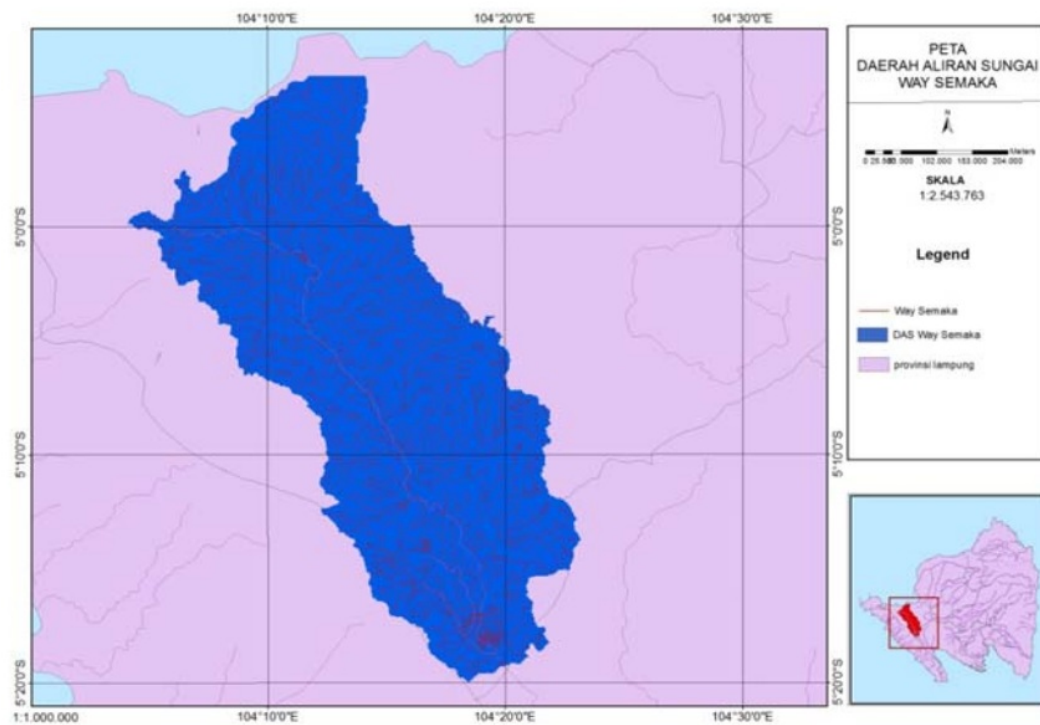
Gambar 6. Jaringan sungai Way Semaka
