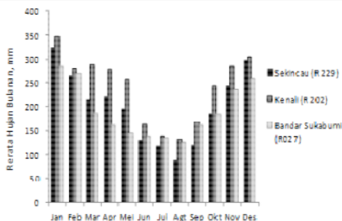
Gambar 2. Hujan rerata bulanan DAS Way Semaka
