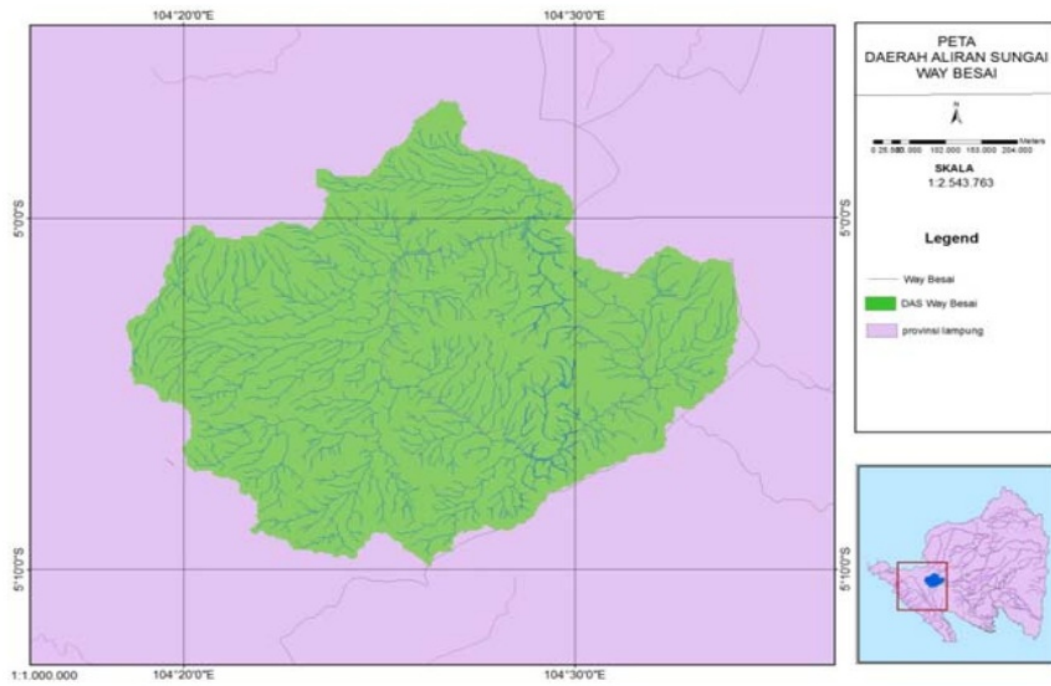
Gambar 5. Jaringan sungai Way Besai
