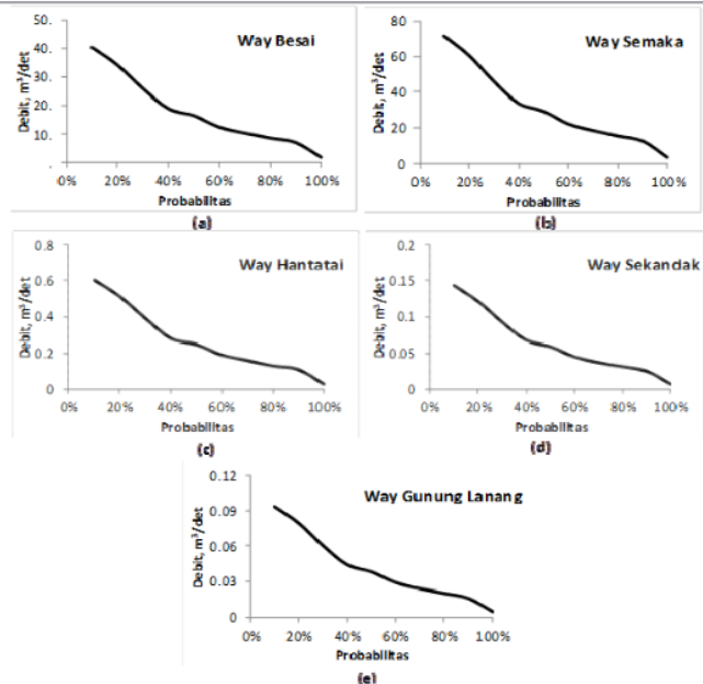
Gambar 7. FDC sungai-sungai (a) Way Besai, (b) Way Semaka, (c) Way Hantatai, (d) Way Sekandak, dan (e) Way Gunung Ratu
