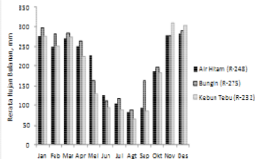
Gambar 1. Hujan rerata bulanan DAS Way Besai
