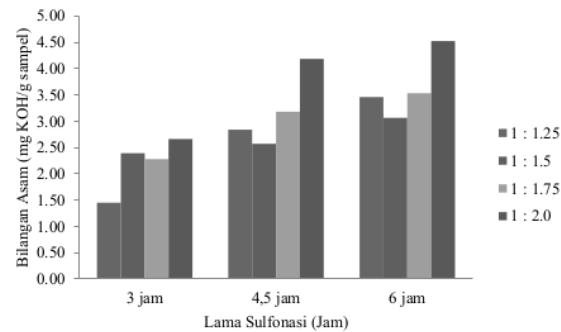
Gambar 6. Pengaruh rasio mol dan lama sulfonasi terhadap bilangan asam pada MES dari metil ester minyak sawit
