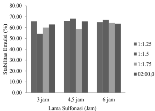
Gambar 4. Pengaruh rasio mol dan lama sulfonasi terhadap stabilitas emulsi pada MES dari metil ester minyak sawit
