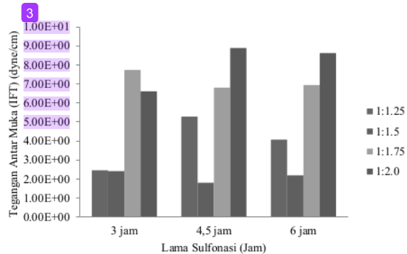
Gambar 3. Pengaruh rasio mol dan lama sulfonasi terhadap IFT pada MES dari metil ester minyak sawit
