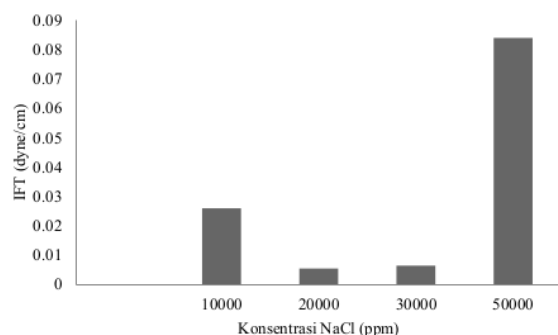
Gambar 9. Pengaruh konsentrasi NaCl terhadap IFT MES
