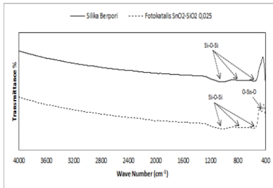
Gambar 4. Spektrum FTIR Fotokatalis SnO 2 -SiO 2 0,025 dan Silika Berpori
