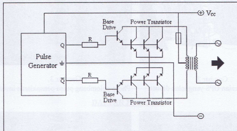
Gambar.1. Rangkaian Utama Sistem Inverter.
