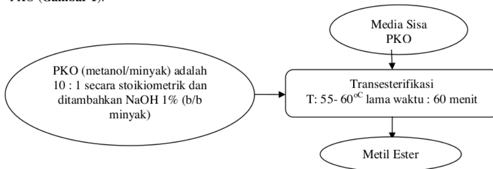
11 Gambar 1. Proses pembuatan metil ester dari minyak inti sawit (PKO) Sumber: Wijayanti, 2008 (yang dimodifikasi)
