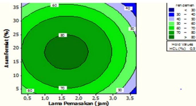
Gambar 6. Kontur respon rendemen sebagai fungsi dari HCl dan asam formiat pada proses pulp TKKS
