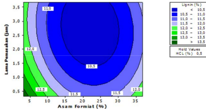
Gambar 4. Kontur respon lignin sebagai fungsi dari asam formiat dan lama pemasakan pada proses pulp TKKS.
