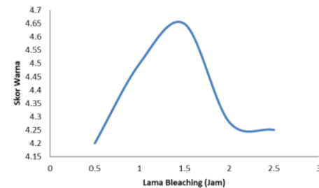
Gambar 4. Pengaruh lama waktu pemutihan terhadap skor warna pulp TKKS
