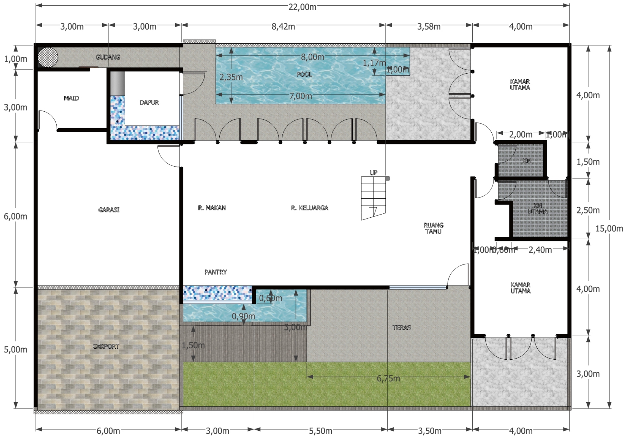
DENAH LT.1
