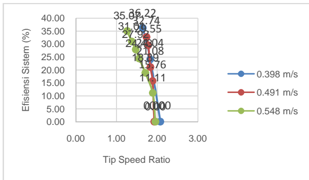
Gambar 6. Grafik hubungan antara tip speed ratio ( ) terhadap efisiensi sistem pembangkit listrik
