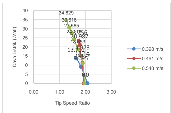
Gambar 5. Grafik hubungan antara tip speed ratio ( ) terhadap daya listrik yang dihasilkan.
