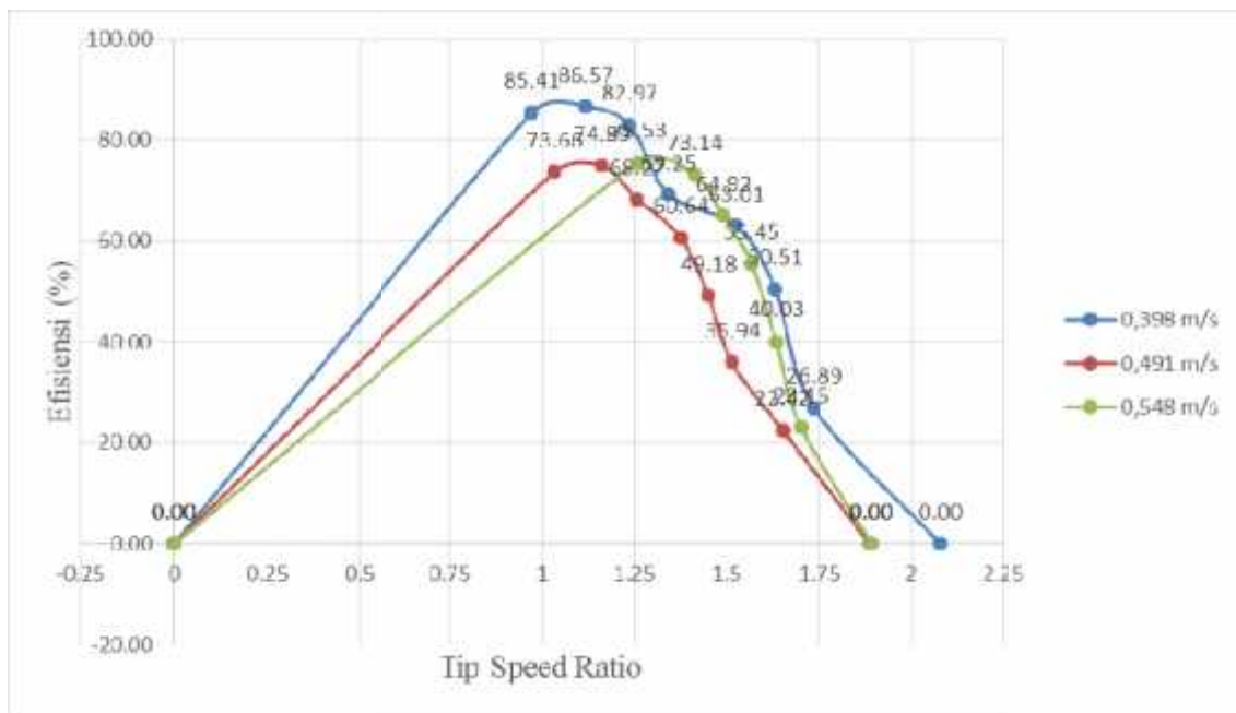
Gambar 7. Grafik hubungan antara tip speed ratio ( ) terhadap efisiensi turbin.
