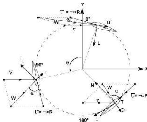
Gambar 1. Diagram kecepatan pada turbin udara sumbu vertikal
