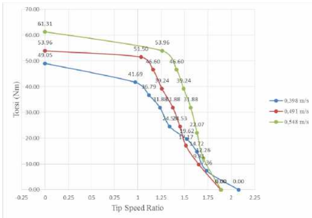
Gambar 5. Grafik hubungan antara tip speed ratio ( ) terhadap torsi yang dihasilkan turbin.
