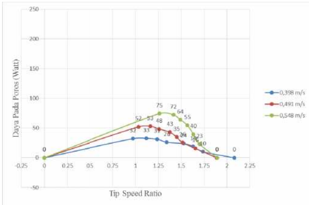
Gambar 6. Grafik hubungan antara tip speed ratio ( ) terhadap daya poros turbin.
