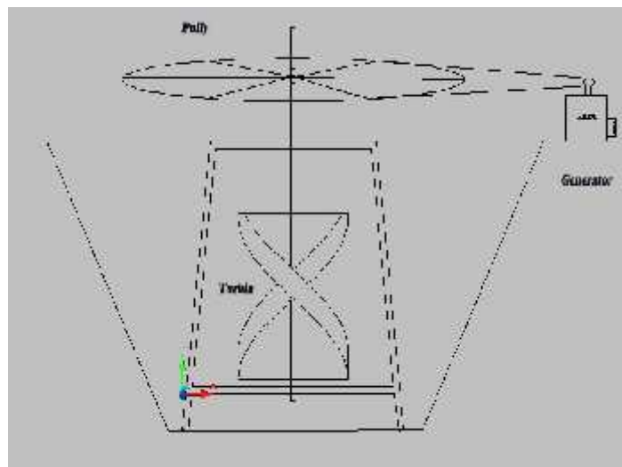
Gambar 2. Skema pengujian turbin helik untuk model sistem pembangkit listrik.
