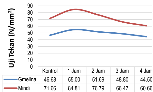
Gbr 5. Grafik uji Tekan
