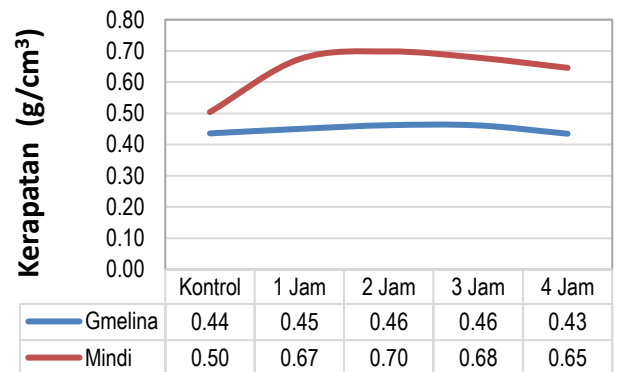
Gbr 4. Grafik perubahan kerapatan sampel kayu
