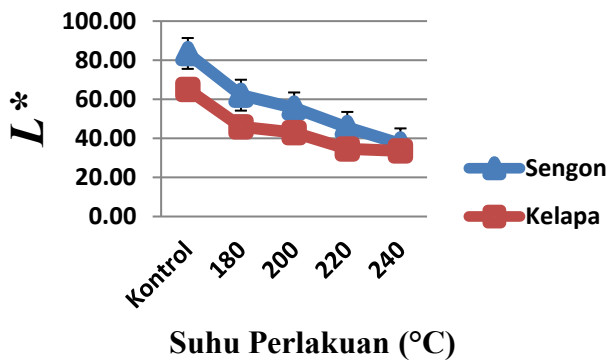
Gbr. 4 Nilai kecerahan ( L^* ) kayu sengon dan kelapa
