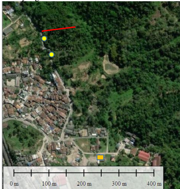
Gambar 2. Lokasi pengamatan lapangan (titik kuning), lintasan survey geolistrik (garis merah) terhadap kantor Kelurahan Pidada (kotak oranye).
