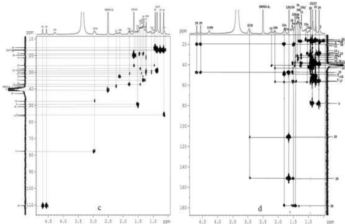
Figure 4. DEPT135 and DEPT90 NMR (a); ^1\text{H} - ^{13}\text{C} HOSY (b); HMQC (c); HMBC spectra (d)
