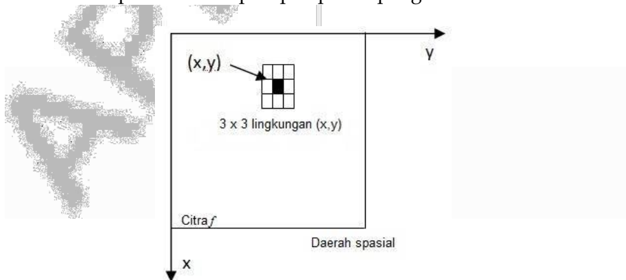
Gambar 3.1 Lingkungan 3×3 dari Sebuah Titik (x,y) pada Citra dalam Daerah Spasial
