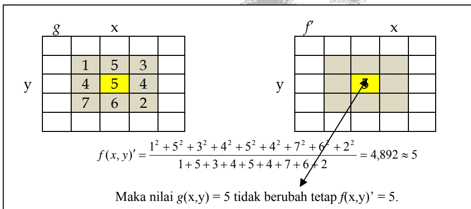
Gambar 4.21 Proses Penghilangan Derau Menggunakan Tapis Rerata Kontraharmonik
