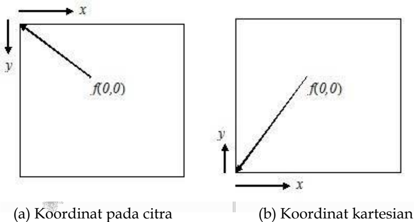
Gambar 1.5 Perbedaan Letak Titik Asal (0,0) pada Koordinat Citra dengan Koordinat Kartesian
