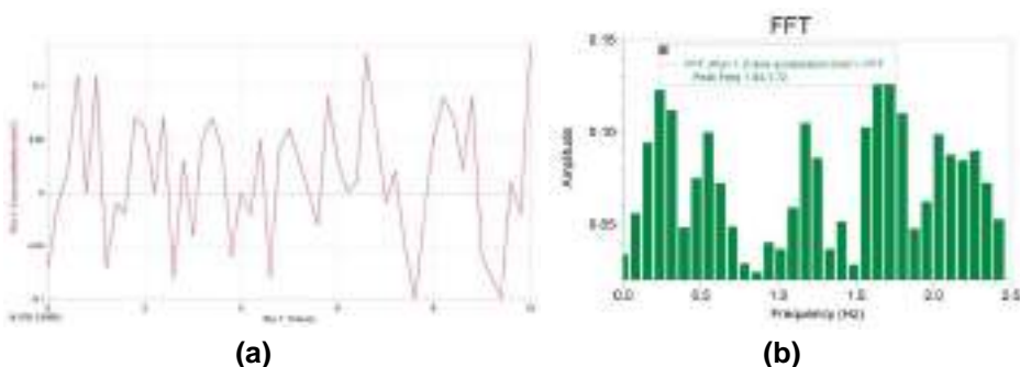
Gambar 6. (a) Getaran orang berjalan seberat 60 kg dalam arah memanjang pelat. (b) Frekuensi pelat akibat orang berjalan arah x dengan berat 60 kg (uji 2)
