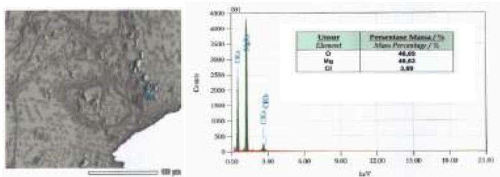
Gambar 11. Grafik Analisis Kualitatif P-Mg 200 \mu\text{m} (Pembesaran 500x)
