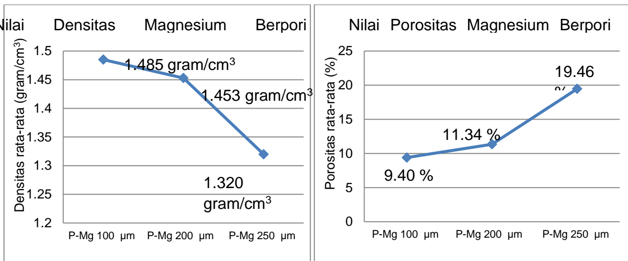
Gambar 6. Grafik Nilai (a). Densitas dan (b) Porositas
