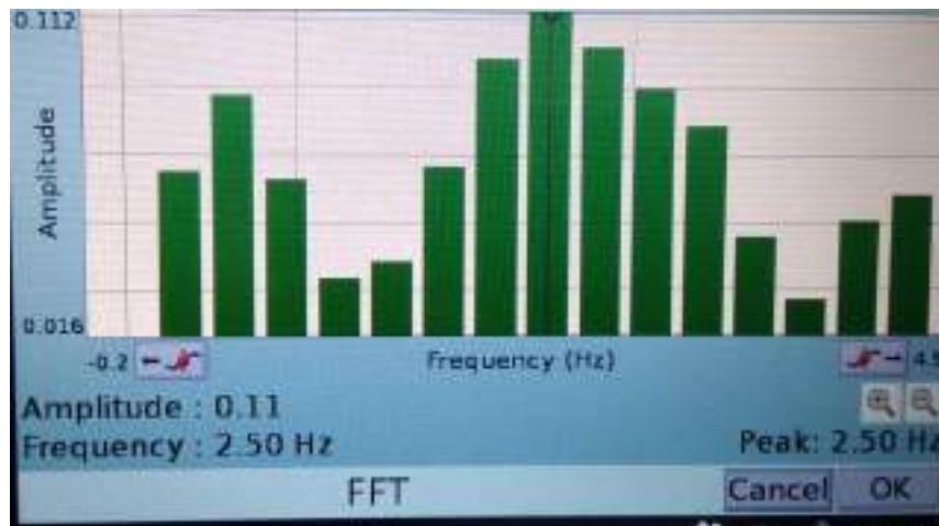
Gambar 10. Analisis FFT untuk pelat yang dibebani oleh 40 orang yang difokuskan pada daerah sekitar diatas balok anak menyilang pada pelat.
