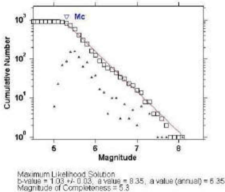
Gambar 5. Nilai a value, b value dan M_c dengan software z-map pada data gempa di sekitar Pulau Ambon
