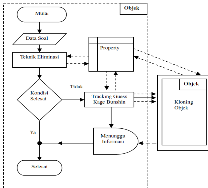
Gambar 3.3. Flow Chart Sebagai Objek Teratas
