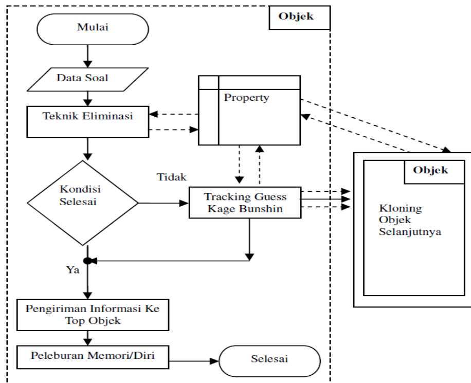
Gambar 3.4. Flow Chart Sebagai Objek Kloning
