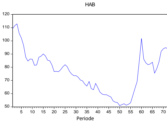
Gambar 2. Plot Data Harga Acuan Batubara (HAB)
