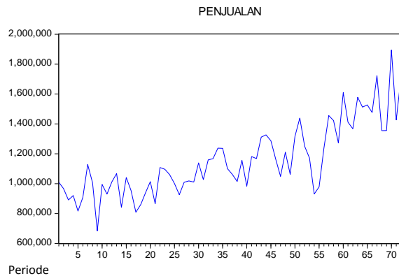
Gambar 1. Plot Data Penjualan Batubara PT. Bukit Asam, Tbk. Unit Pelabuhan Tarahan
