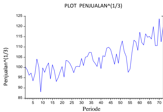
Gambar 5. Plot Data Transformasi Penjualan Batubara
