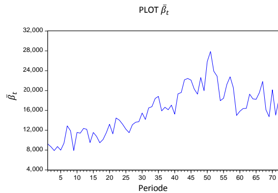
Gambar 3. Plot \bar{\beta}_t Bulan Januari 2012 - Desember 2017
