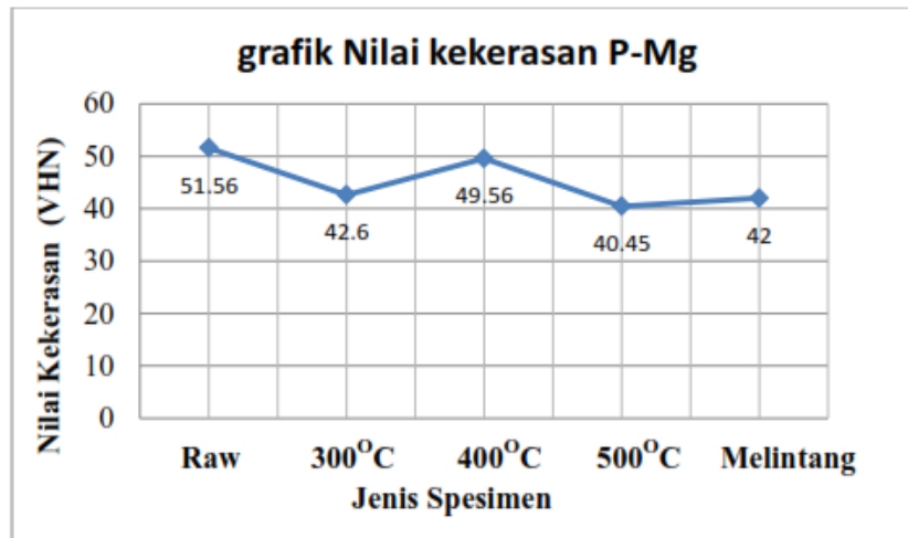
Gambar 11. Grafik kekerasan magnesium berpori, Raw material, P-Mg 300°C, 400°C, dan 500°C dalam posisi melintang
