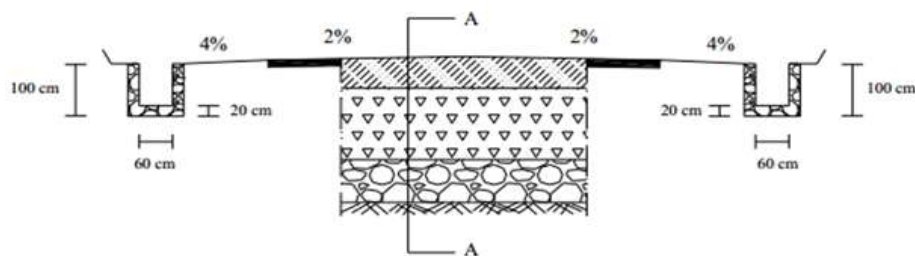
Gambar 4. Penampang melintang
