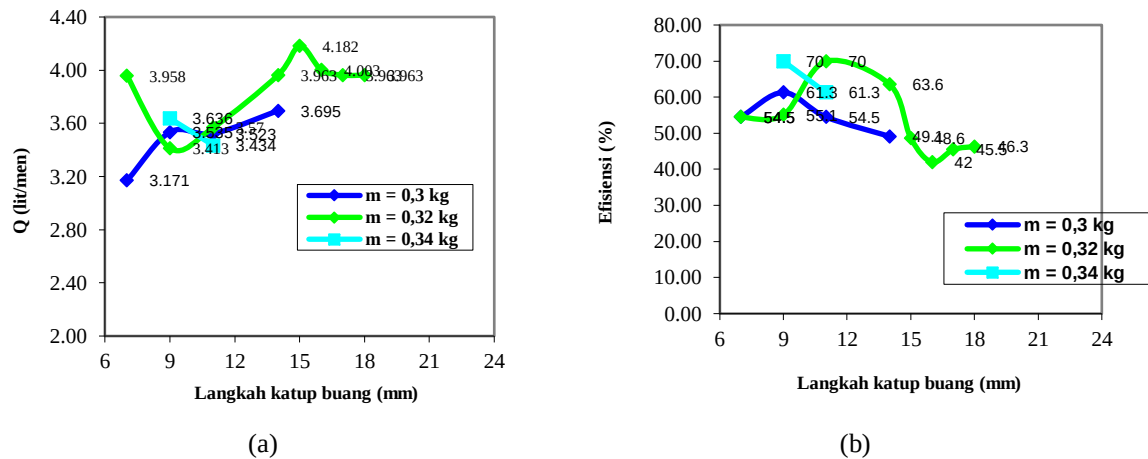
Gambar 1. (a) Grafik hubungan antara laju aliran volume air yang dipompakan terhadap panjang langkah, (b) Grafik hubungan antara efisiensi terhadap panjang langkah katup buang.
