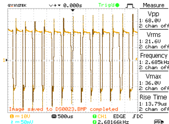
Gambar 12. Keluaran Inverter beban Resistor 10 kOhm
