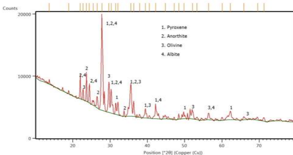
Gambar 1. Hasil analisa XRD batuan basalt Mataram Baru, Lampung Timur
