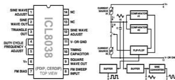
Gambar 4. Rangkaian Skematik pembangkit gelombang sinus
