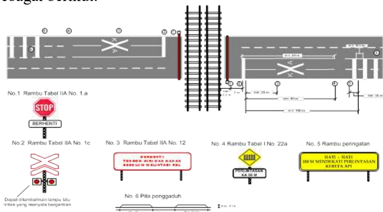
Gambar 3. Kelengkapan Rambu di Perlintasan Berpintu Jalur Ganda
