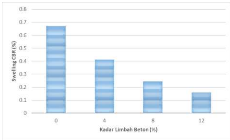
Gambar 2. Hubungan Penambahan Limbah Beton Terhadap Uji Swelling CBR
