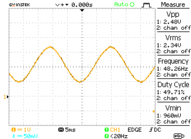
Gambar 6. Hasil Pembangkit Gleombang Sinus
