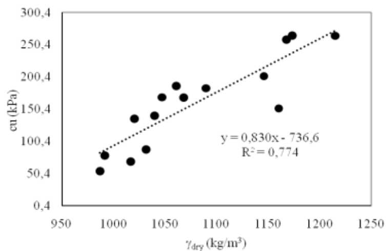
Gambar 5. Grafik Hubungan Antara cu dengan Berat Volume Tanah Kering, \gamma_{dry}
