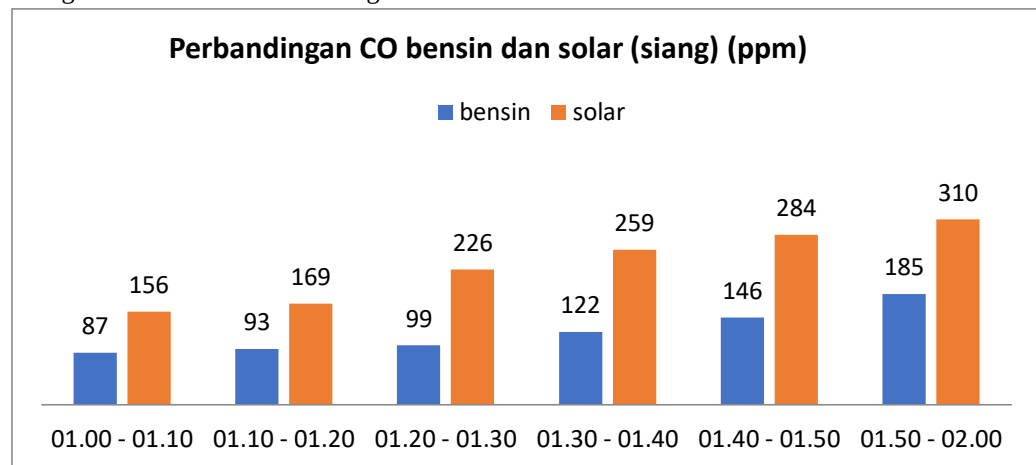
Gambar 5. Perbandingan CO Bensin dan Solar Siang
