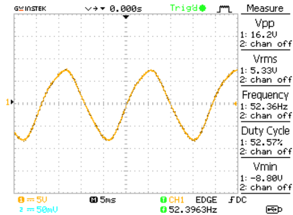
Gambar 16. Output inverter sisi primer terminal 9 Volt
