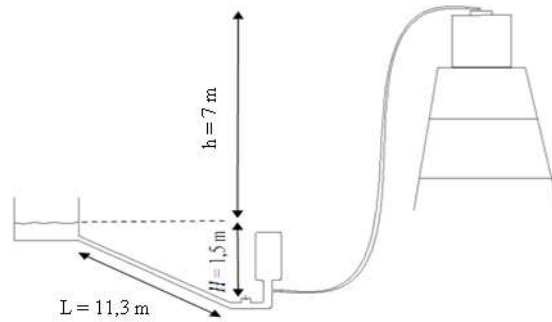
Gambar 4. Skema pemasangan pompa di lapangan
