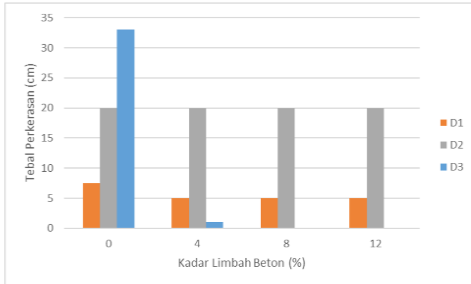
Gambar 3. Hubungan Penambahan Limbah Beton dengan Tebal Lapis Perkerasan
