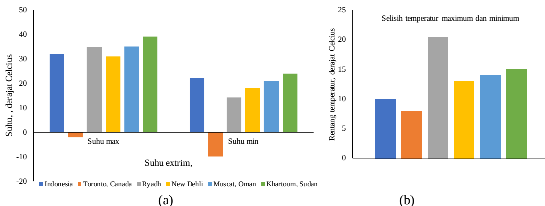
Gambar 3. (a) Temperatur ekstrim, (b) Selisih temperatur ekstrim
