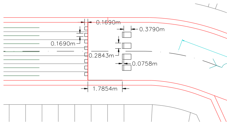
Gambar 3. Desain Kolam Olak BH. 364
