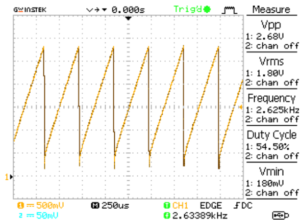
Gambar 9. Hasil Pembangkit gelombang segitiga
