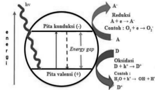
Gambar 5. Mekanisme Fotokatalis [28]
