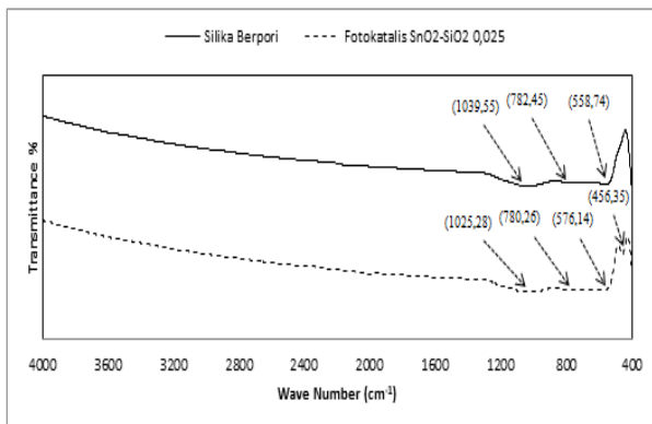
Gambar 4. Spektrum FTIR Fotokatalis \text{SnO}_2\text{-SiO}_2 0,025 dan Silika Berpori
