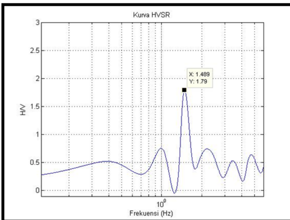
Gambar 8. Kurva HVS
