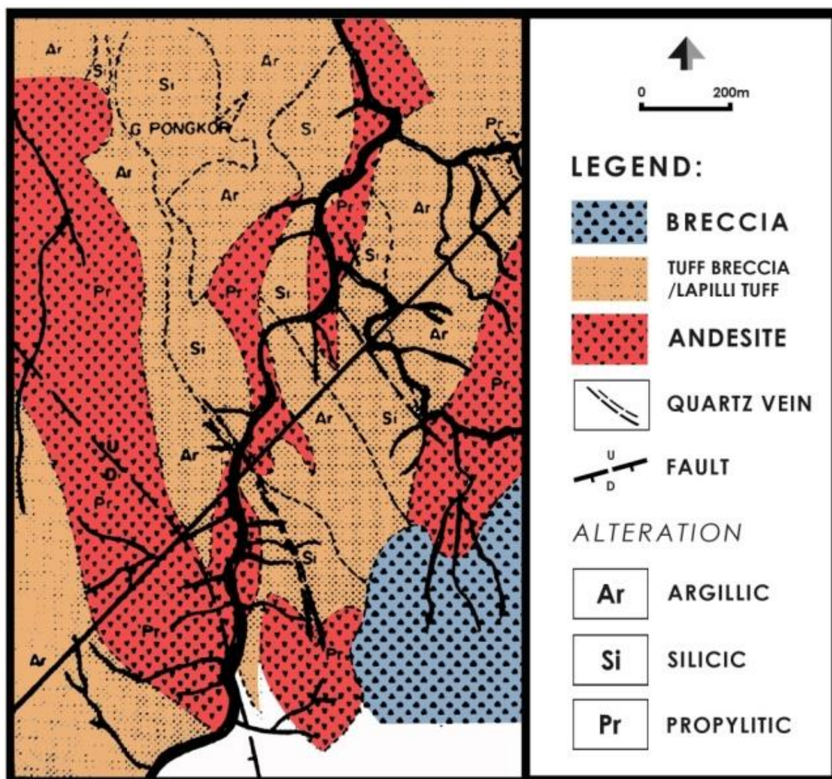
Gambar 1. Peta Geologi Area Gunung Pongkor, dari NE ke SW (Dimodifikasi dari Basuki, dkk., 1994)
