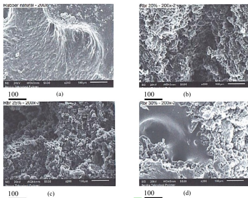
17 Figure 2. SEM Micrograph of NR/CB Composites: (a) NR (b) NR/CB20 (c) NR/CB25 (d) NR/CB30
