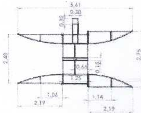
Gambar 4. Ukuran saluran pengarah
