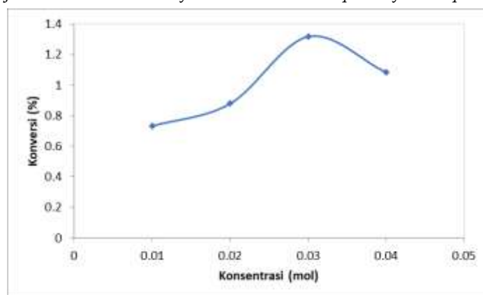
Gambar 3. Pengaruh konsentrasi katalis terhadap konversi \alpha -terpineol
