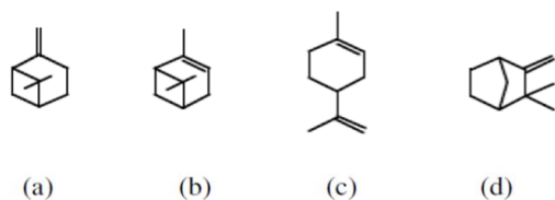
Gambar 1. Struktur senyawa minyak terpentin (a) \beta -pinene, (b) \alpha -pinene, (c) limonene , dan (d) camphene
