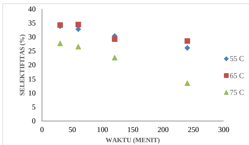
Gambar 11. Hubungan suhu dan waktu reaksi terhadap selektifitas \alpha -terpineol.
