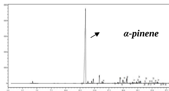
Gambar 7. Grafik Hasil Analisis GC Minyak Terpenin
