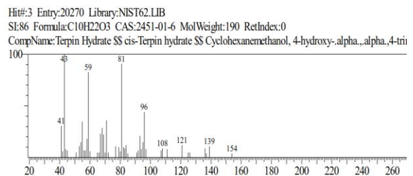
Gambar 10. Hasil Spektrum massa pada peak ke-30
