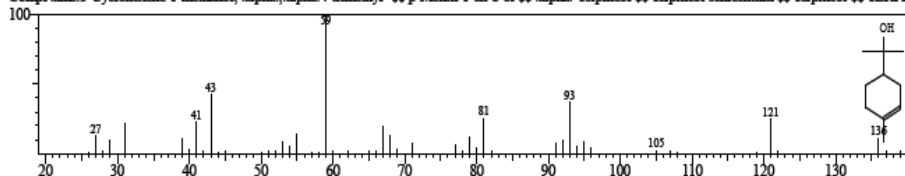
Gambar 13. Hasil spektrum massa pada peak ke-18
