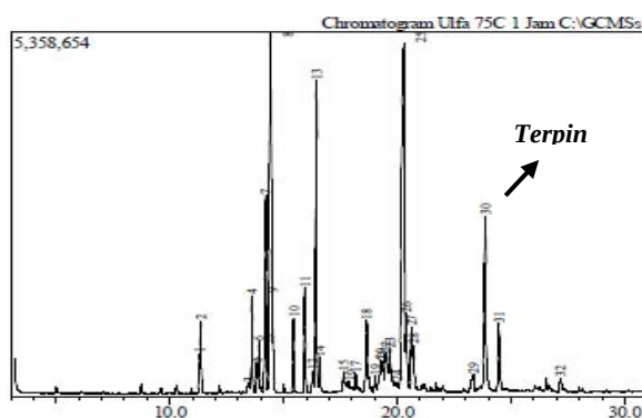
Gambar 9. Hasil Analisis GC-MS Pada Suhu 75°C
