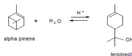
Gambar 2. Reaksi Pembentukan \alpha - Terpineol dari \alpha - Pinene
