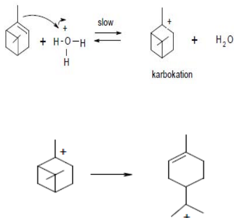
Gambar 3. Adisi Elektrofilik
