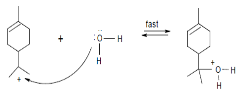
Gambar 4. Adisi Nukleofilik
