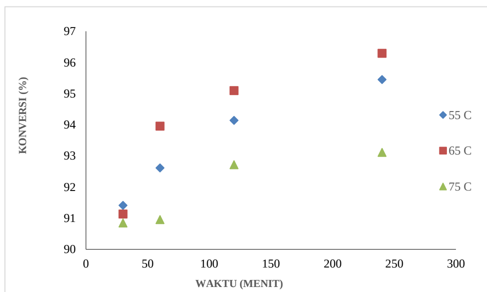
Gambar 8. Hubungan suhu dan waktu reaksi terhadap konversi \alpha -pinene
