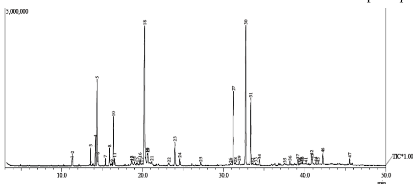
Gambar 12. Hasil analisis GC MS pada suhu 65°C dan waktu reaksi 60 menit
