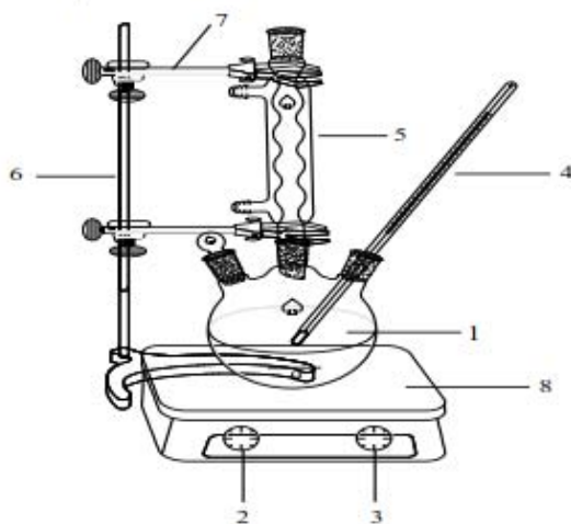
Gambar 6. Alat distilasi untuk reaksi sintesis \alpha -terpineol
