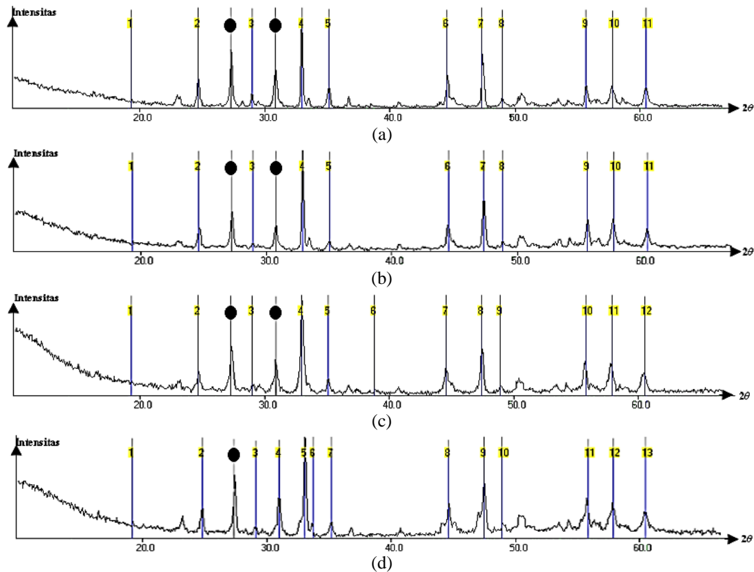
Gambar 1. Hasil analisis XRD dengan program celref ; (a) BSCCO-2223-850, (b) BSCCO-2223-855, (c) BSCCO-2223-860 dan (d) BSCCO-2223-865. Tanda ( ● ) menunjukkan impuritas BSCCO-2212.
