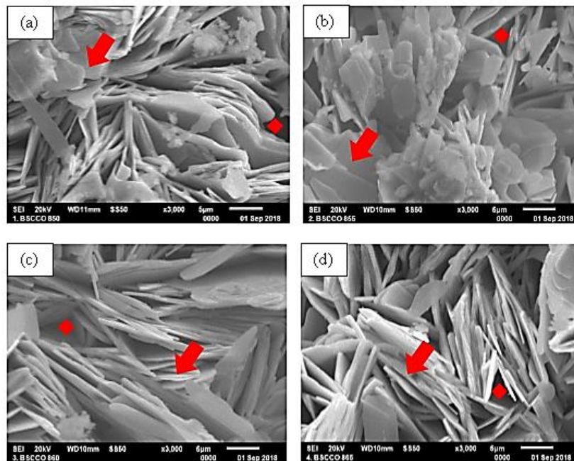
Gambar 2. Hasil karakterisasi SEM pada sampel; (a) BSCCO-2223-850, (b) BSCCO-2223-855, (c) BSCCO-2223-860 dan (d) BSCCO-2223-865 dengan perbesaran masing-masing 3000x. Ket: tanda panah (↴) menunjukkan lempengan yang telah terorientasi, dan tanda (◆) menunjukkan void.
