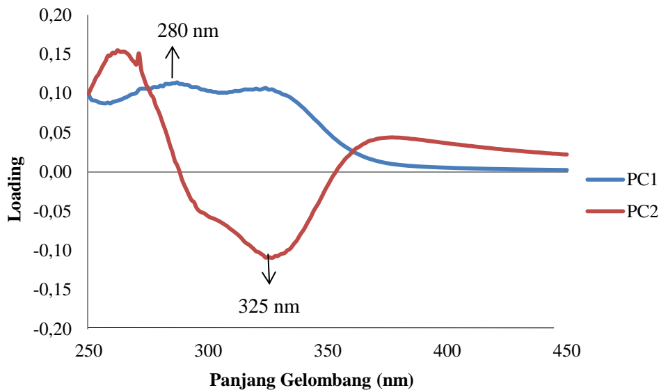
Gambar 4. Nilai X-Loading PC1 dan PC2
