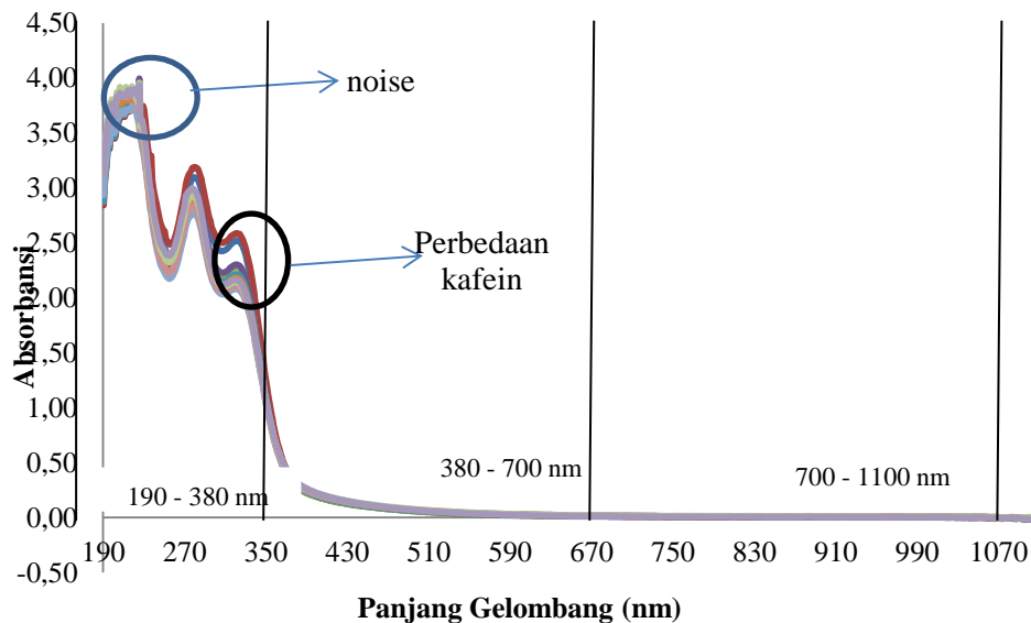
Gambar 1. Spektra 200 Sampel Campuran Kopi Dekaf - Non Dekaf pada Panjang Gelombang 190-1100 nm.
