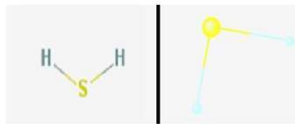
Gambar 1. Struktur Kimia Hidrogen Sulfida 10
